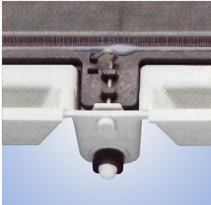
Verschluss und Gummistopfen für Reinigungsbügel
