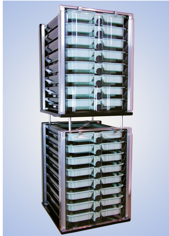
C0013350 16er-Brutschrank Forelle mit transparenter Frontabdeckung und Wasserablaufwanne
